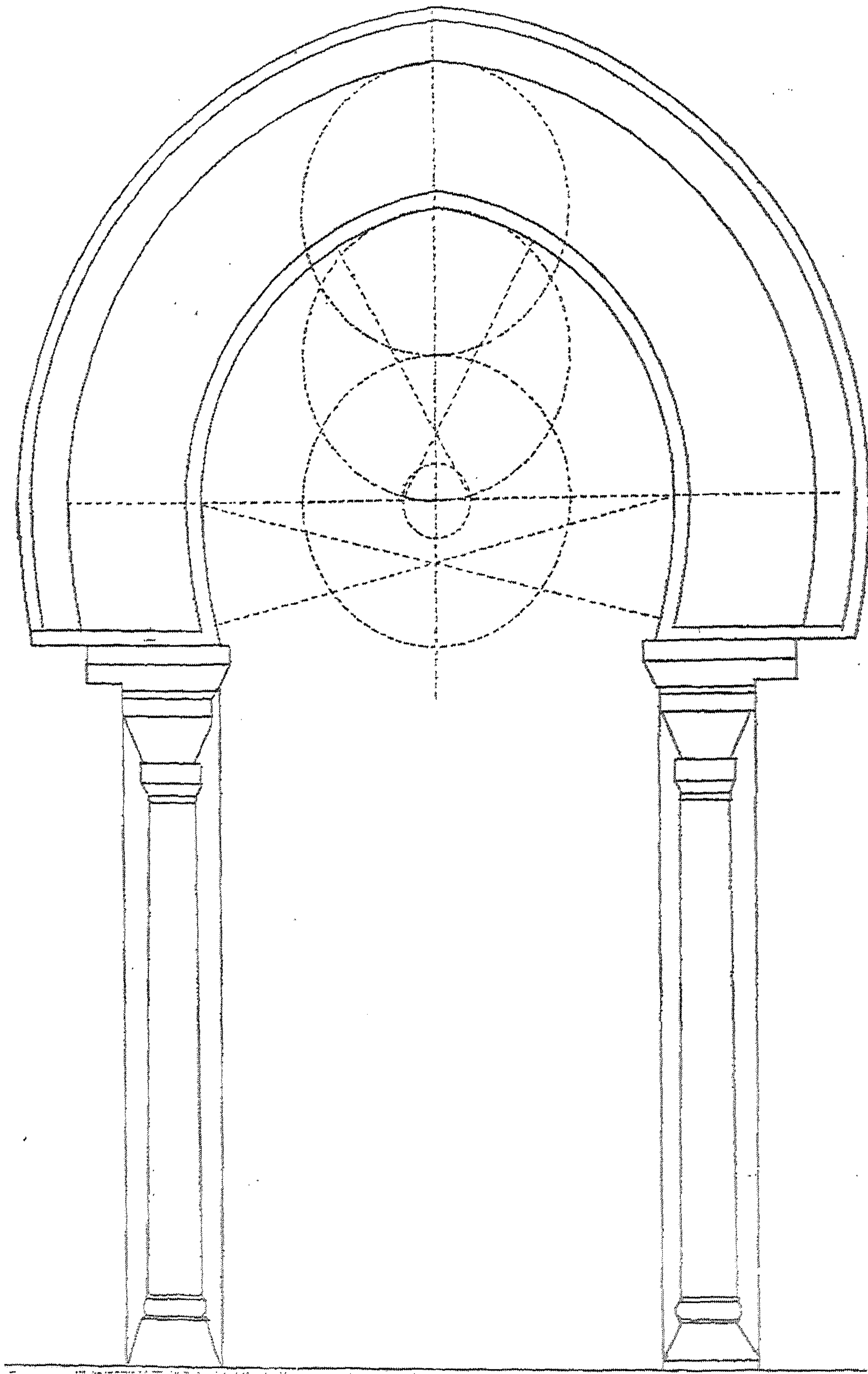
(شكل رقم ٢٥) رسم للعقد المحيط بمحراب جامع القيروان عن جولفان
